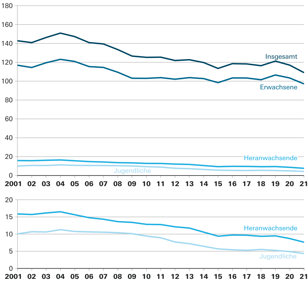
Abb. 1 Rechtskräftig Verurteilte in Bayern seit 2001 nach Altersgruppen in Tausend
